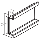
TH35-7.5 DIN rail
