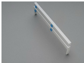
32964 000 Seitenmodul für Sammelschienenadapter beidseitig ansteckbar 9 x 200 für: EMC60..
