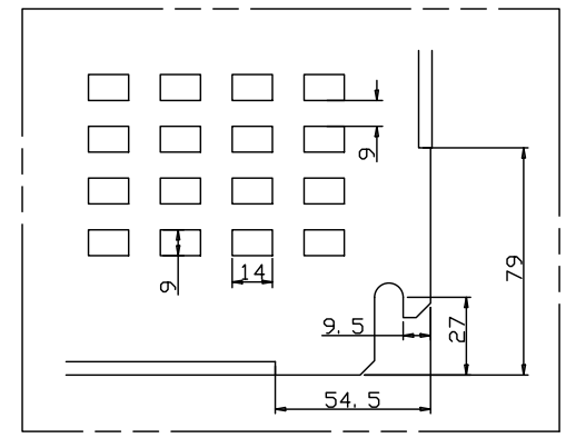
DETALLE X
