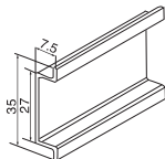
TH35-7.5 DIN Rail
