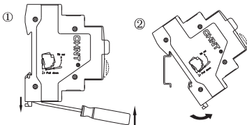
TH35-7.5 DIN Rail
