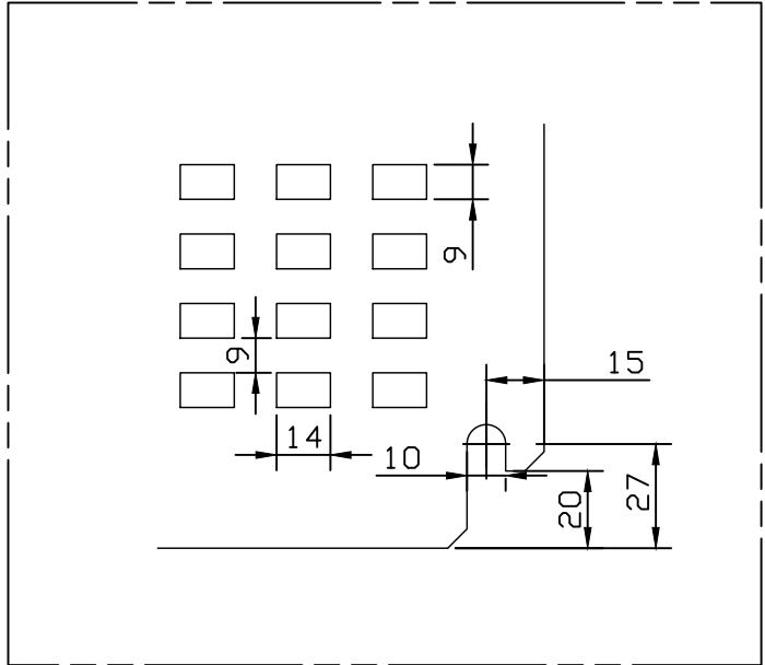
DETALLE X
